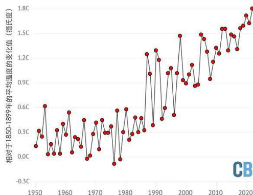
六月份创纪录高的陆地温度
